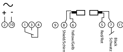
Abb. 2 Schaltschema CA-D
